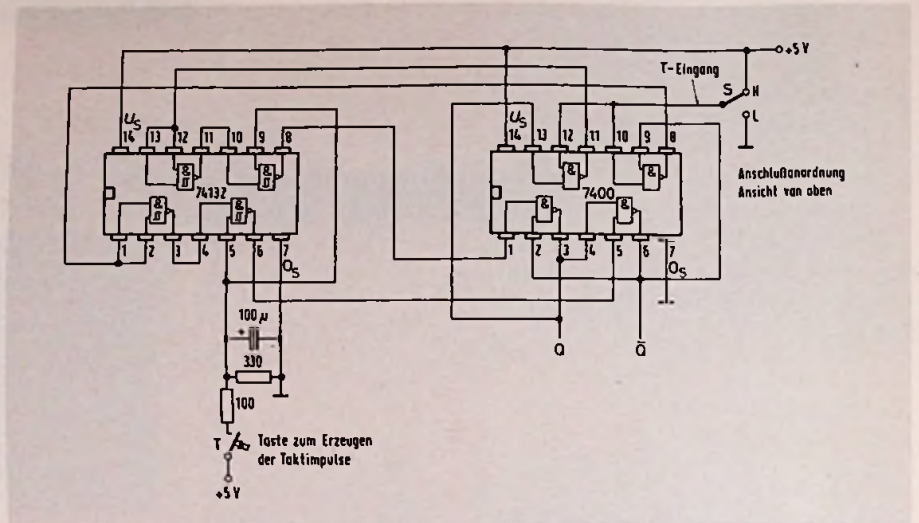
Bild 15.3.2. Experimentier-Aufbau für ein T-Flip-Flop aus NAND-Gliedern
