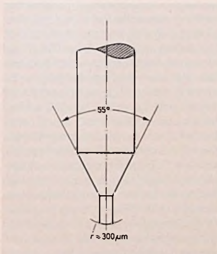
Bild 3. Pathé-Abtastnadel für Schallplatten mit Tiefenschrift
