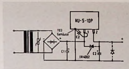
Bild 2. Der Regler NU-5-10P kann unmittelbar auf das Kühlblech geschraubt werden, da sein Gehäuse an Masse liegt
