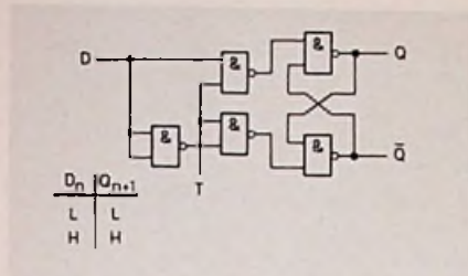
Bild 15.2.2. D-Flip-Flop aus NAND-Gliedern und Wahrheitstabelle des D-Flip-Flops
