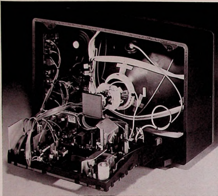
Bild 2. Statt vieler kleine Moduln enthält das Profi-Compact-Chassis zwei Groß-Moduln, die in der Werkstatt repariert werden können
