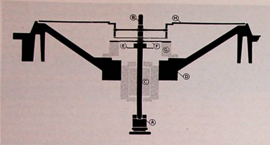
Bild 3. Schnitt durch Teller und Antrieb der Schallplatten-Wiedergabe-Maschine EMT 950. A Stützlager, B Tellerzapfen an der Hauptwelle, C Rotor des Motors, D verripptes Gußchassis, E Tachoscheibe mit Präzisionsteilung, F Bremmscheibe für Schnellstopp, G Bremsmagnet, H Epoxyharz-Teller mit 33 cm Außendurchmesser
