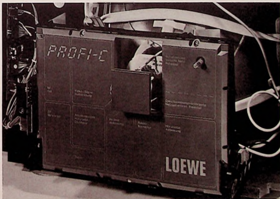
Bild 1. Die Abdeckkappe gibt dem Profi-Compact-Chassis zusätzlichen Halt
