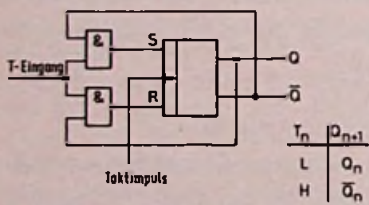
Bild 15.3.1. T-Flip-Flop und Wahrheitstabelle. Ein T-Flip-Flop entsteht durch Rückführung der Ausgangssignale auf zwei UND-Gatter, die als Datenweiche arbeiten
