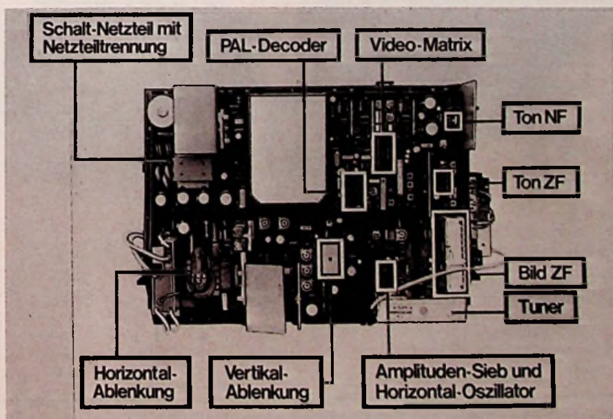
Bild 3. Der Chassis-Groß-Modul enthält bis auf die Fernbedienschaltung alle Baugruppen vom Tuner bis zum Netzteil
