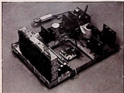
Ablenkeinheit und Stromversorgung dieses Fernseh-Chassis arbeiten nach dem Cessy-T-Konzept (ITT)
