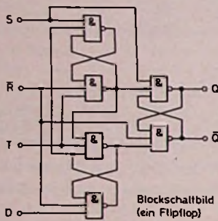
Bild 15.2.3. Innenschaltung des 2fach D-Flip-Flops 7474
