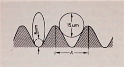
Bild 5. Abtastverhalten von konischer und elliptischer Abtastnadel
