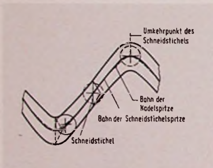
Bild 4. Die unterschiedliche Form von Schneidstichel und konischer Abtastnadel ist Ursache für nichtlineare Verzerrungen
