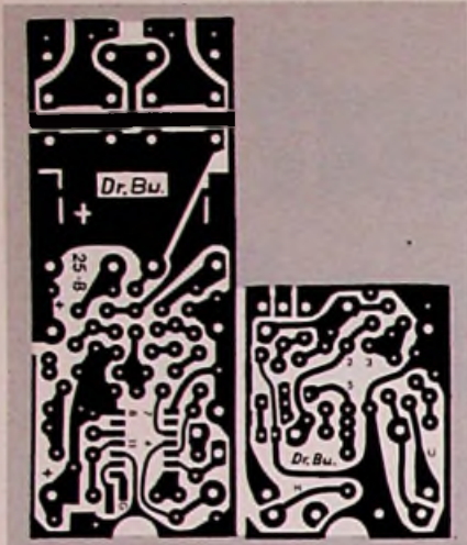
Bild 10. Platinen des Pilotschalters II im Maßstab 1 : 1. Netzteil siehe Bild 6 in Heft 9 S. T 444
