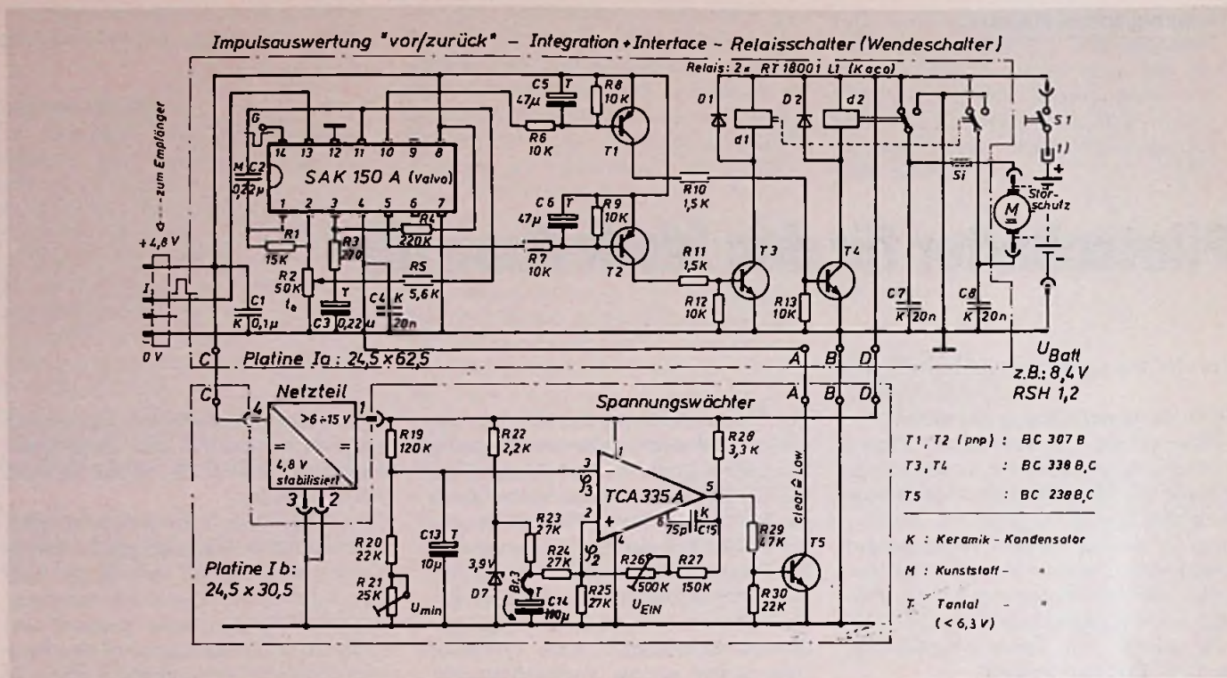
Bild 8. Schaltung des Pilotschalters II für Reversierbetrieb mit Spannungswächter. Netzteil wie in Bild 3
