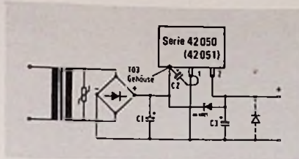
Bild 1. Einige Spannungsregler kann man wegen ihrer Pin-Belegung unmittelbar gegen einen Transistor im TO-Gehäuse austauschen
