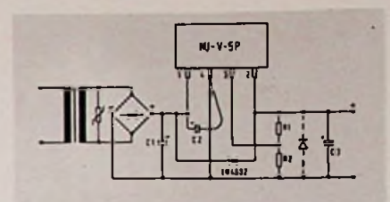
Bild 3. Einstellbarer Regler mit vier Anschlüssen und isoliertem Aufbau (Bilder: Nucletron Vertriebs GmbH, München)
