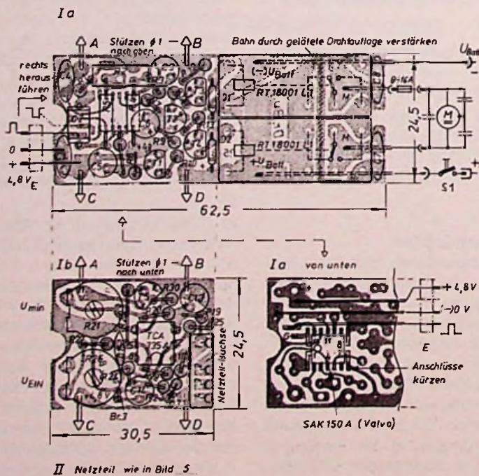
Bild 9. Bestückungsplan des Pilotschalters II, Netzteil siehe Bild 5 in Heft 9
