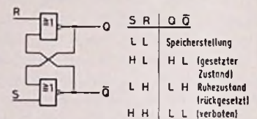
Bild 15.1.4. Schaltung des NOR-Flip-Flops und seine Wahrheitstabelle
