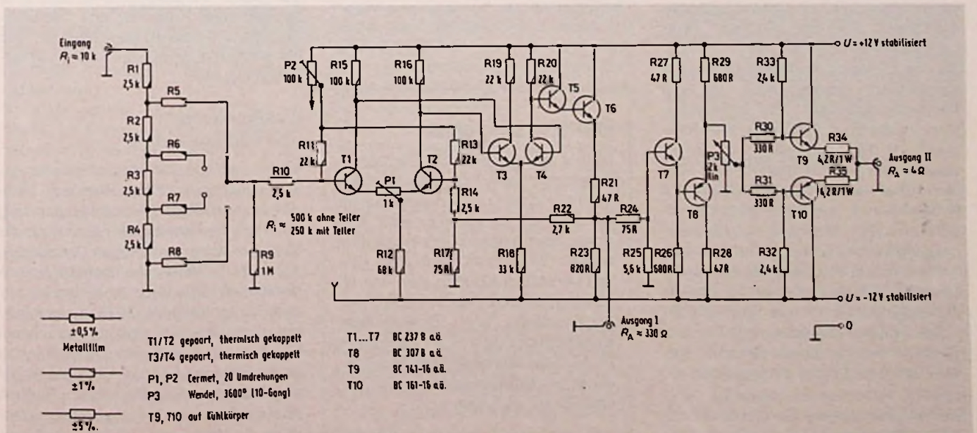
Bild 1. Schaltbild des Meßverstärkers. Der mit einem Pfeil versehene Anschluß von Potentiometer P2 wird mit der -12-V-Sammelschiene verbunden. Der Wert der Widerstände R32 und R33 muß 6,8 \text{ k}\Omega sein statt 2,4 \text{ k}\Omega .
